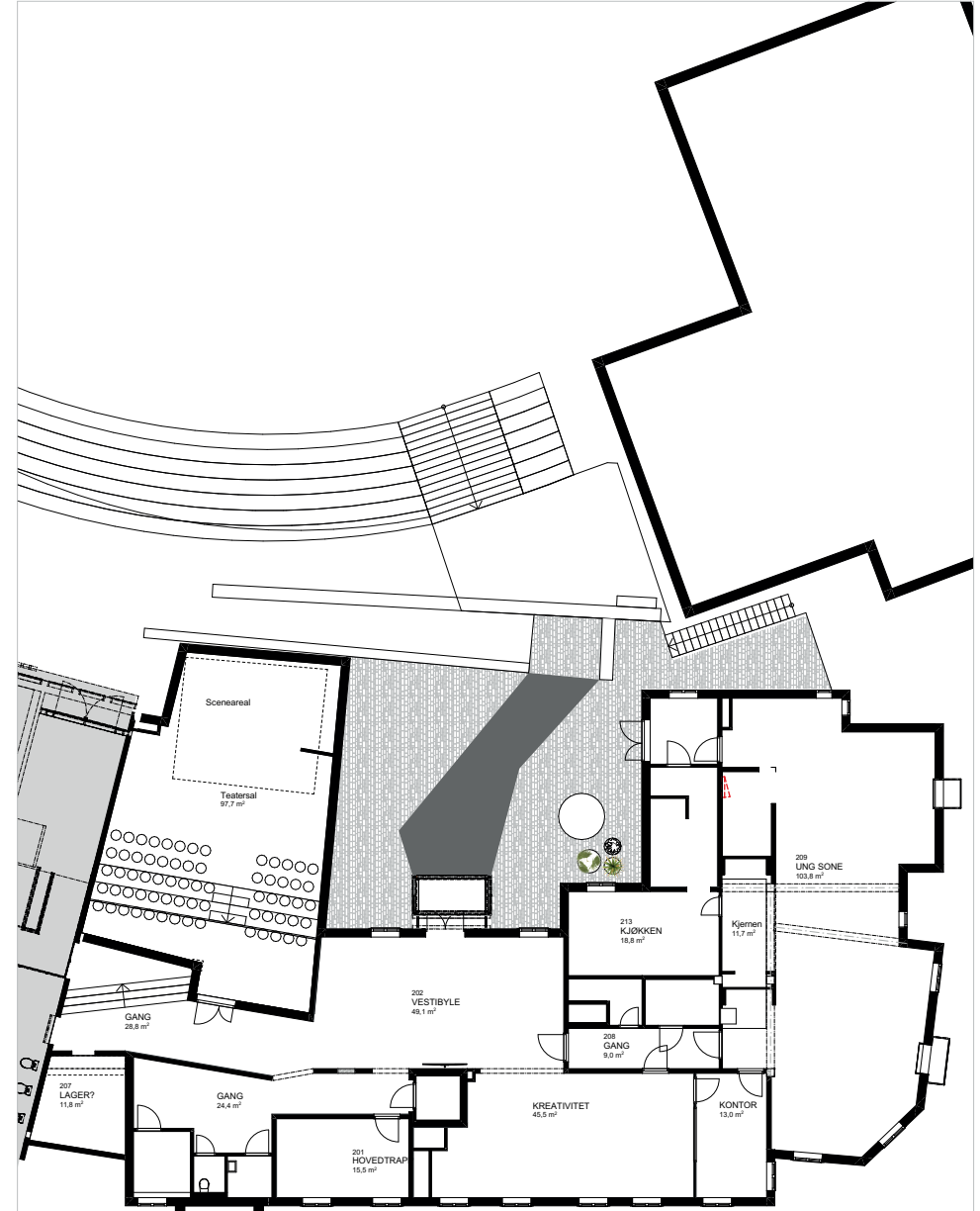
Utsnitt plan 2. etasje
